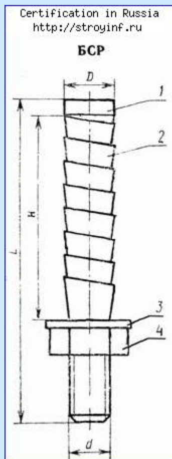
1-болт; 2-ЗЭ; 3-шайба; 4-гайка
