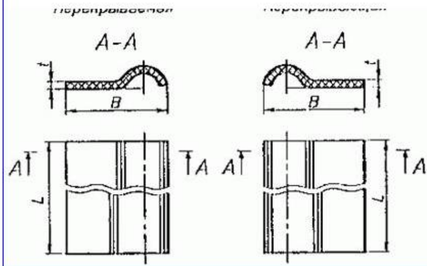
Рисунок 3-Упрощенные коньковые детали
