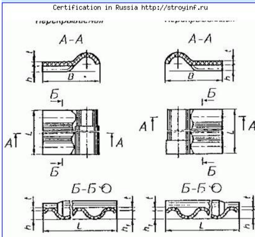
Рисунок 2-Коньковые детали
