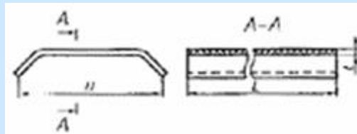
Рисунок 5-Лотковая деталь
