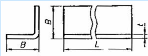
Рисунок 4-Равнобокая угловая деталь
